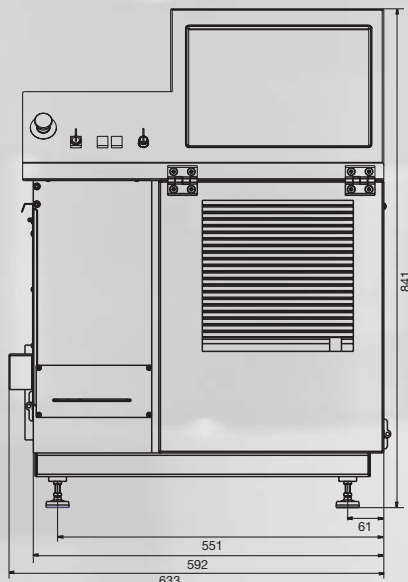
Vorderansicht
